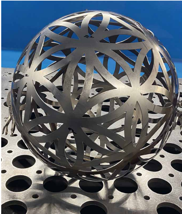
«Lichtkugel» geschweisste Halbschalen, Ausschnitt mit 3D Laser
